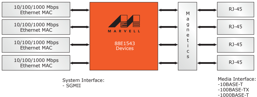
图 1: SGMII 至铜缆应用
