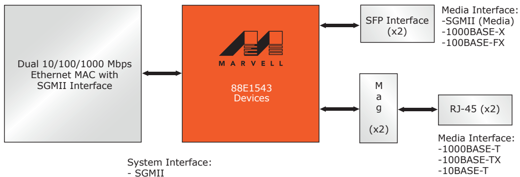
图 2: 带 AutoMedia 的双端口 SGMII (系统) 至铜缆/SGMII/光纤
